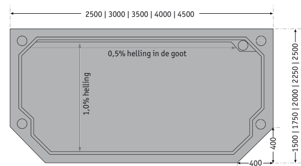
Zeshoekige plattegrond
