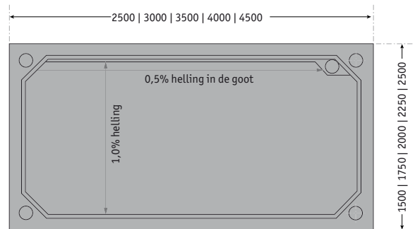
Rechthoekige plattegrond
